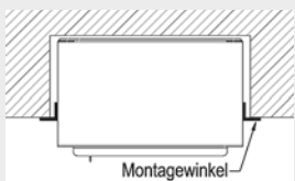
Montagevariante C / Variante C (mit Montagerahmen / avec équerre)
