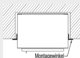
Montagevariante C / Variante C (mit Montagerahmen / avec équerre)
